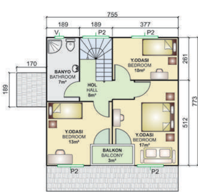
56 m 2 + 3 m 2 = 59 m 2 1.Kat Planı / First Floor Plan
