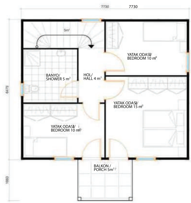
Üst Kat Planı / First Floor Plan 56 m 2
