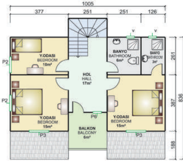
66 m 2 + 6 m 2 = 72 m 2 1.Kat Planı / First Floor Plan
